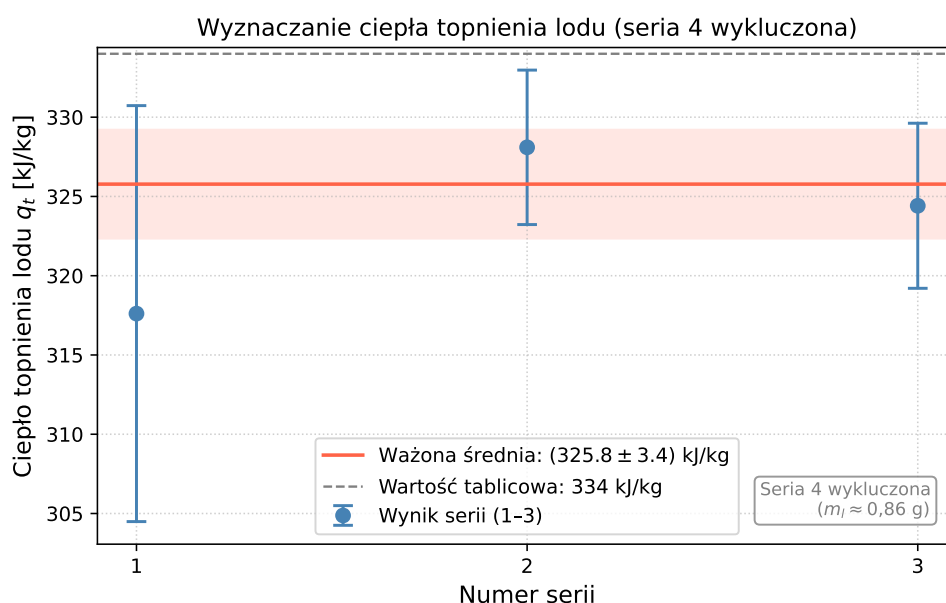
Rysunek 2: Wyznaczone ciepło topnienia lodu dla serii 1–3 z niepewnościami pomiarowymi. Linia czerwona — ważona średnia (??); pasmo — jej niepewność; linia szara przerywana — wartość tablicowa 334 \text{ kJ kg}^{-1} . Seria 4 ( m_l \approx 0,86 \text{ g} ) została wykluczona.
